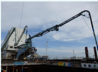
コンクリートミキサー船
