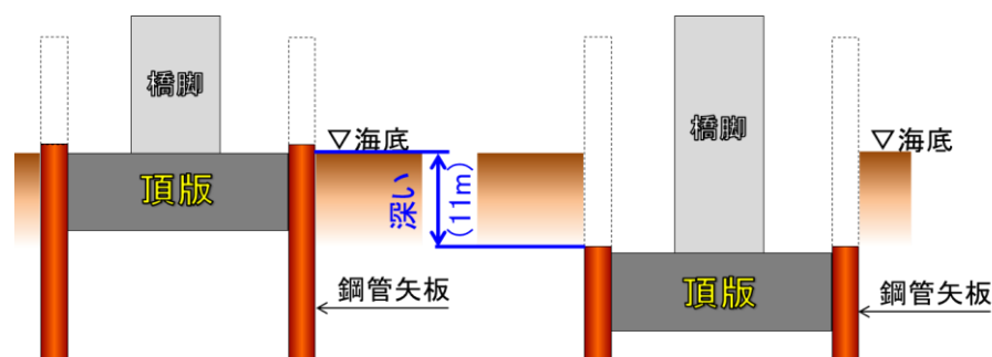
一般的な鋼管矢板井筒基礎
